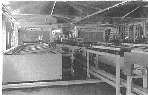
更新した高周波プレス機(レゾ、8径プレス)
